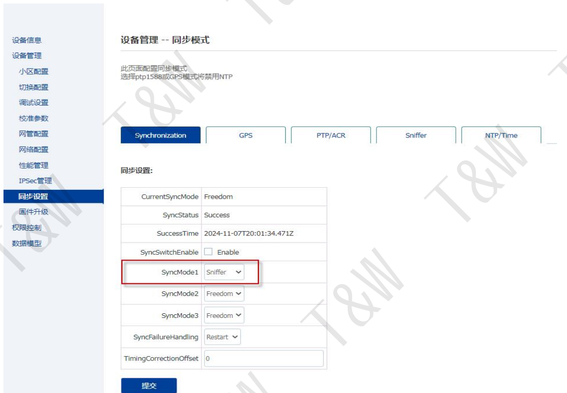
图 30: Sniffer 同步配置
