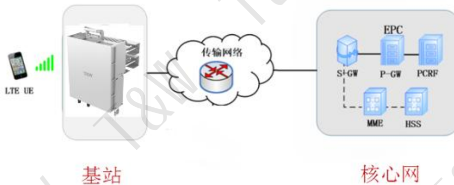
图 2：网络组网基站直连核心网
