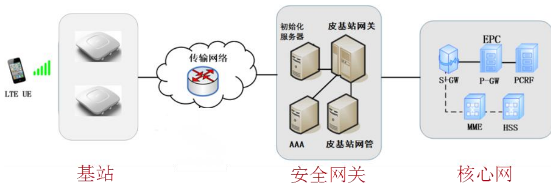
图 1：网络组网带安全网关
